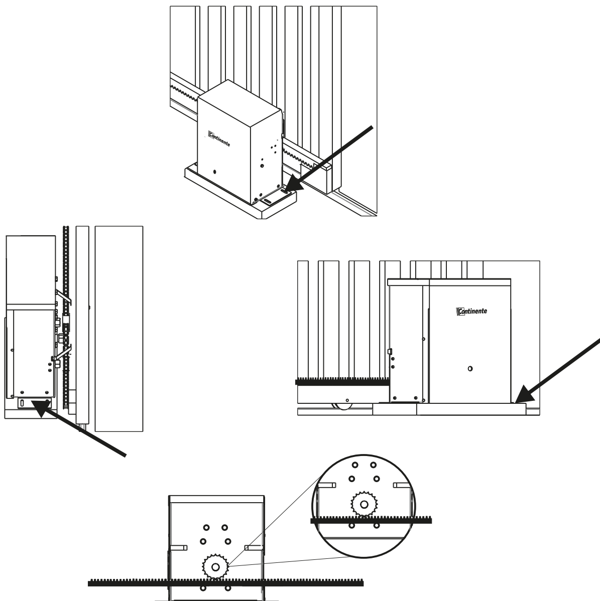
Figura 01: Fixar as base do Movimentador Deslizante
